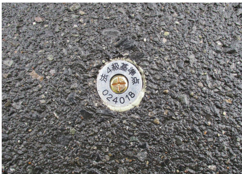
<道路地内に設置された4級基準点の例>
