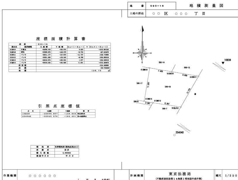
<地積測量図>
