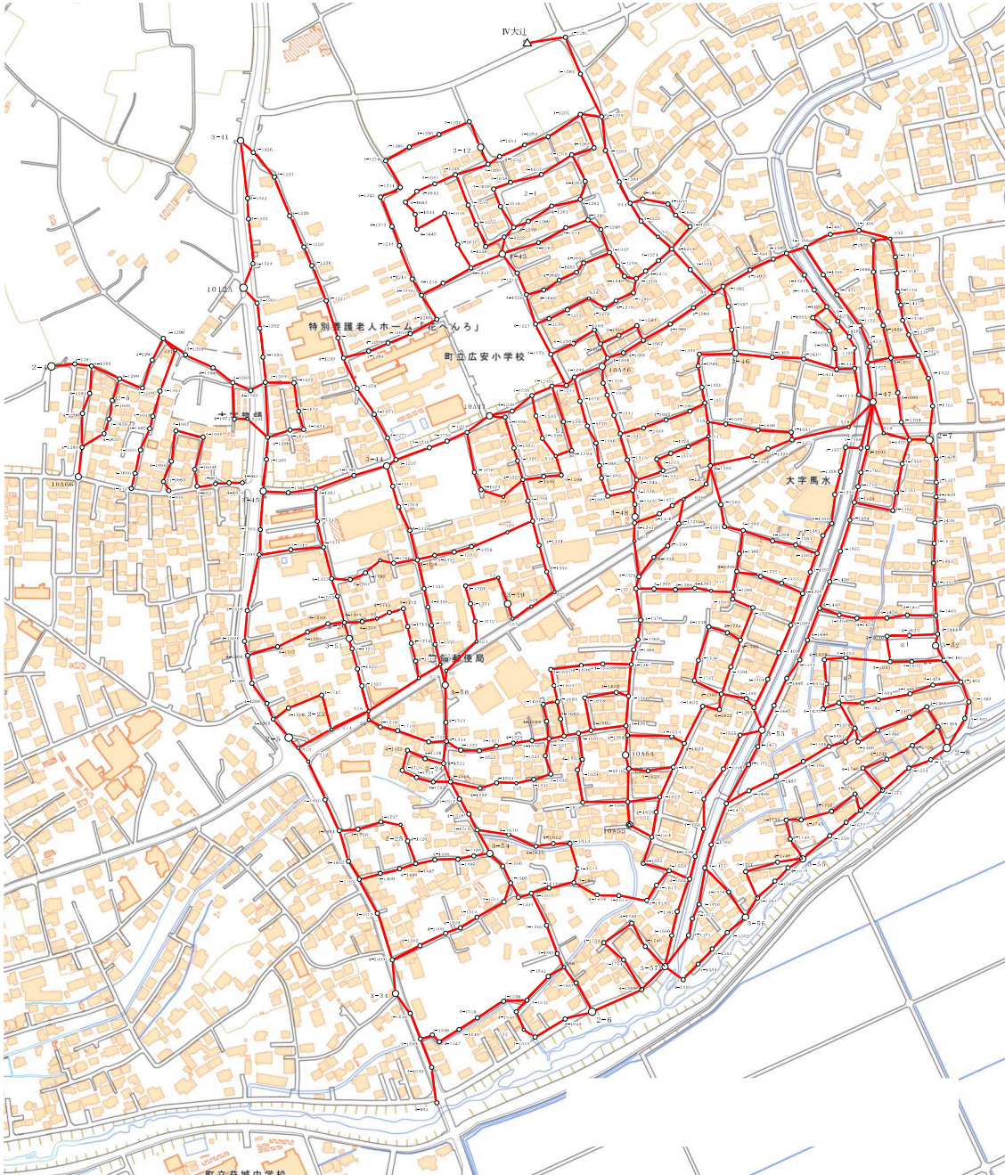
令和4年度 上益城郡益城町惣領ほか地区 4級基準点 網 図
